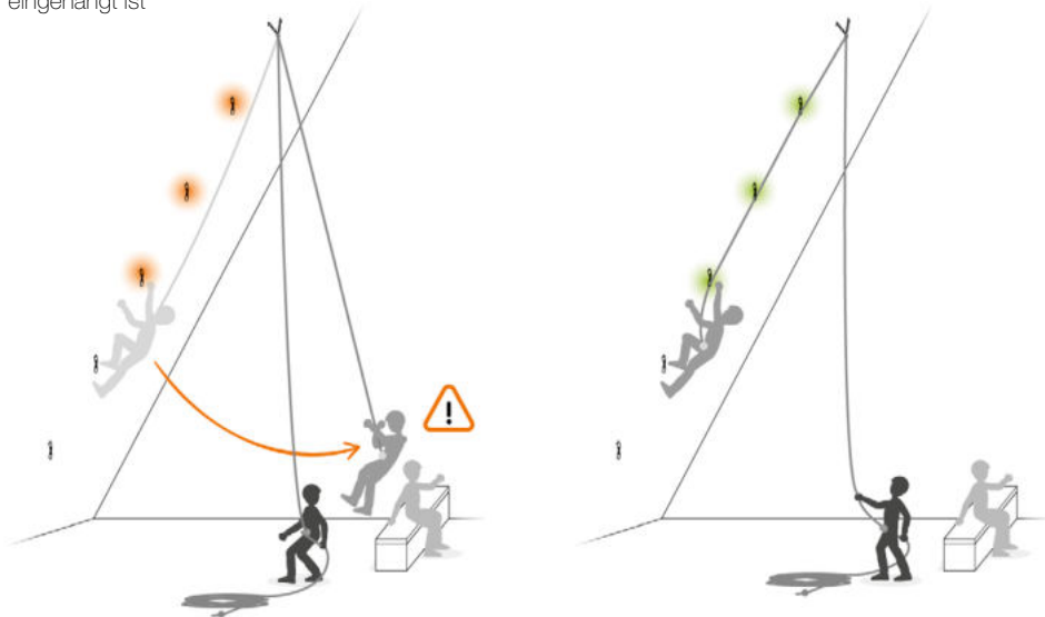
Im Überhang: Am Seilstrang klettern, der in die Zwischensicherungen eingehängt ist
